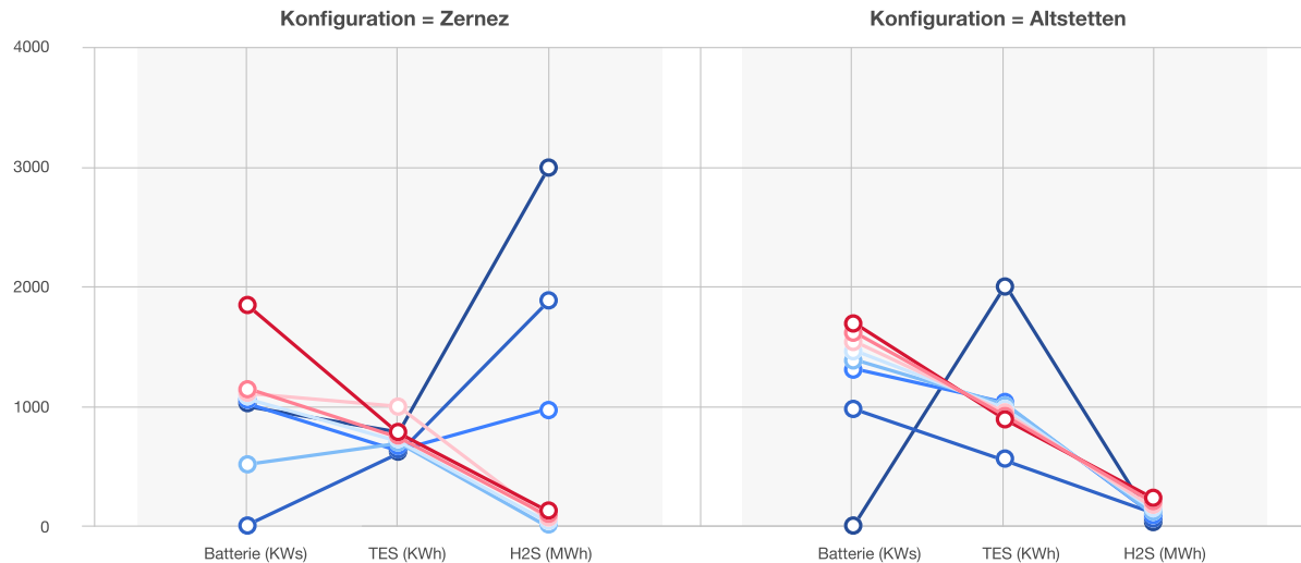
Abbildung 5. Umfang der untersuchten Speichertechnologien (Batterie, thermische Warmwasserspeicherung, H 2 -Speicherung) für Zernez (links) und Altstetten (rechts) für eine Mehrzieloptimierung, welche die jährlichen Gesamtkosten (Rottöne) und die CO 2 -Emissionen (Blautöne) minimiert.
