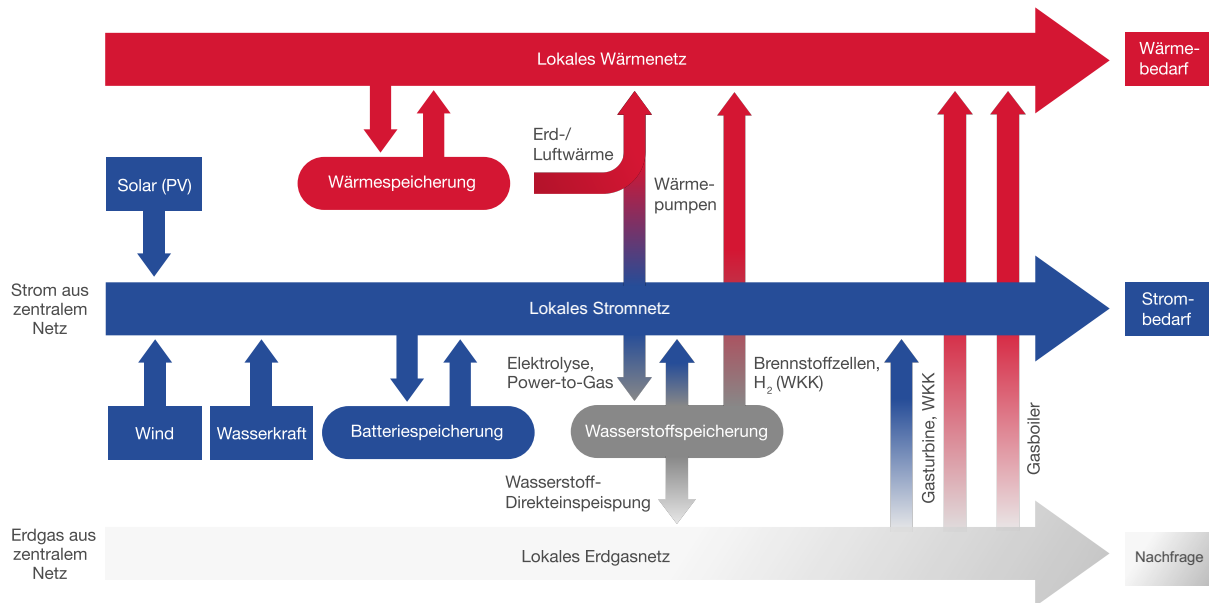
Schematische Darstellung eines DMES. Quelle: Projekt «Dezentrale Energiesysteme»
